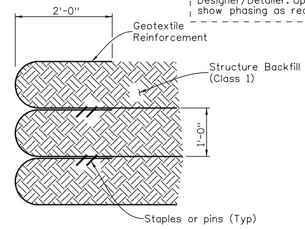
WRAP DETAIL
