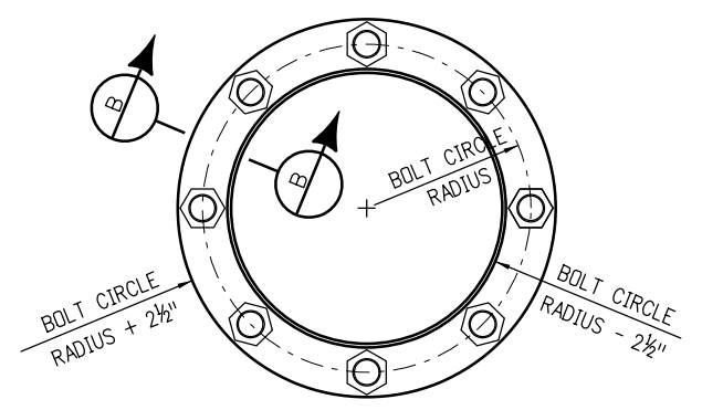
Bolt Template
